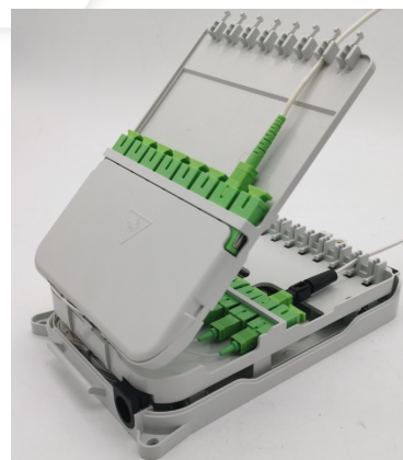
Soporta 16 conectores SC
