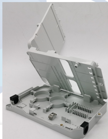
Diseño incluye 2 bandejas
